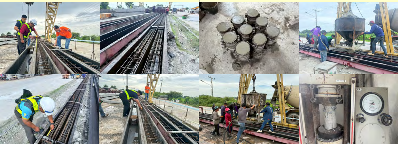
งานหล่อเสาเข็มคอนกรีตอัดแรง ขนาด 0.22x0.22 ม. และขนาด 0.26x0.26 ม.
